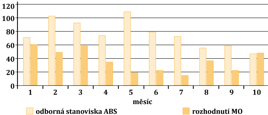
Srovnání počtu odborných stanovisek ABS a rozhodnutí MO v roce 2013
